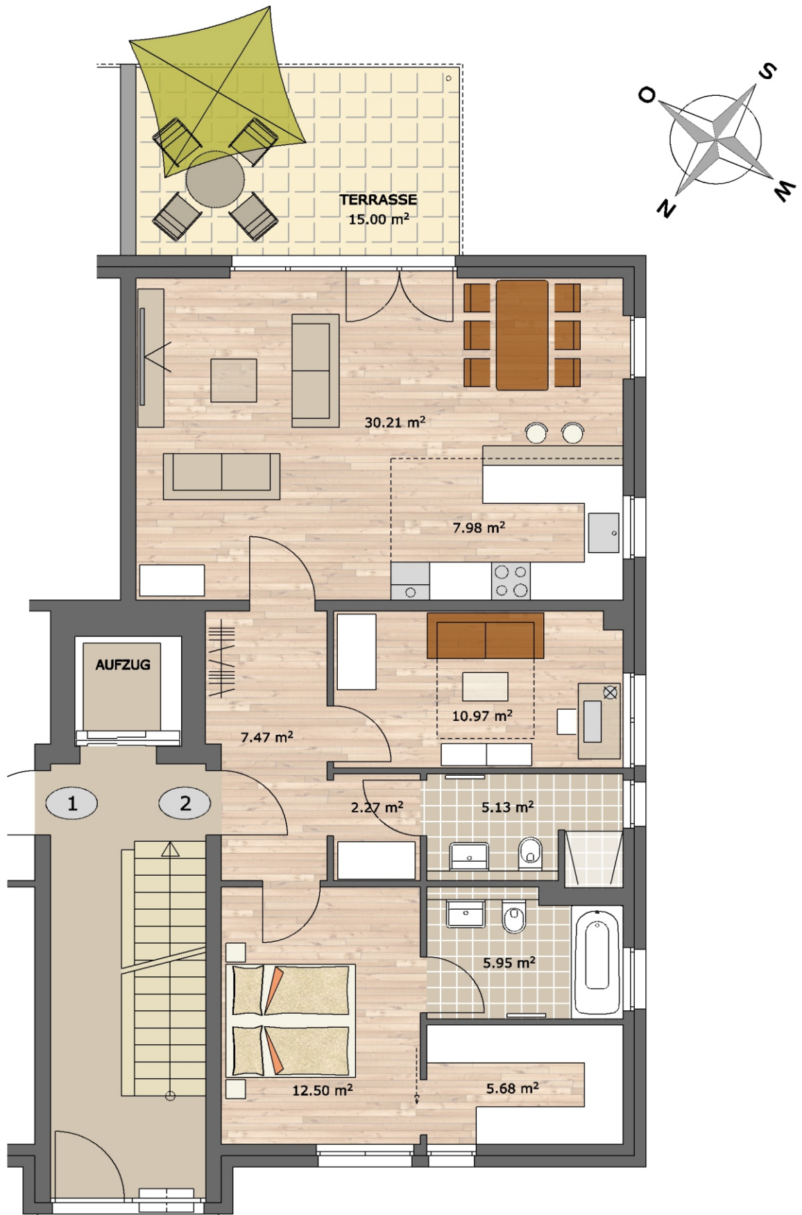
VOGELSANGSTR. 144 ERDGESCHOSS 3-ZIMMER 96 m 2
